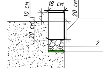
Схема установки бортового камня вдоль внутридворовых автомобильных проездов бордюры 1000*300*180
