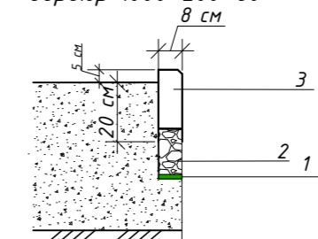
Схема установки бортового камня на пешеходных дорожках и площадках бордюры 1000*200*80
