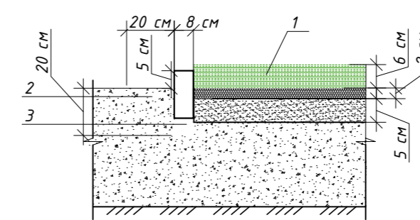
Схема покрытия газона (тип 3)
